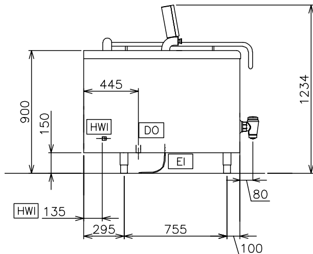
Zij aanzicht
